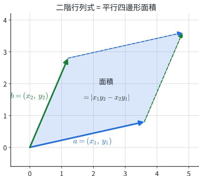
圖 3-5：以 \vec{a} = (x_1, y_1) 、 \vec{b} = (x_2, y_2) 為鄰邊的平行四邊形，其面積等於二階行列式的絕對值 |x_1 y_2 - x_2 y_1| 。
