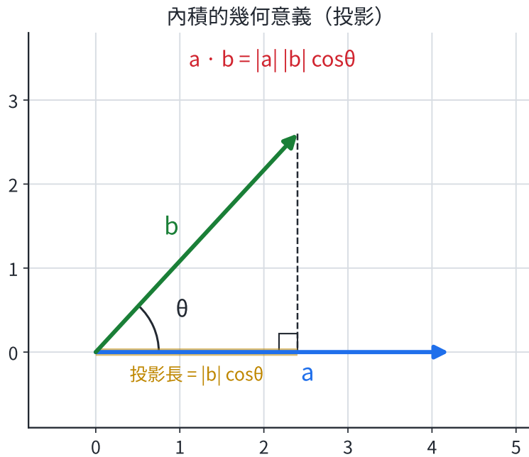
圖 3-3：內積的幾何意義。 \vec{b} 在 \vec{a} 方向上的投影長為 |\vec{b}| \cos \theta ，乘上 |\vec{a}| 即得內積 \vec{a} \cdot \vec{b} = |\vec{a}| |\vec{b}| \cos \theta 。
