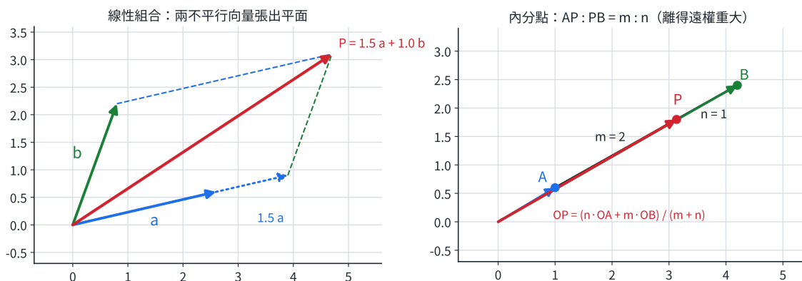
圖 3-2：左——線性組合，以兩個不平行向量 \vec{a} 、 \vec{b} 為基底，調整係數 s 、 t 即可張出（拼出）平面上任一向量 P = s\vec{a} + t\vec{b} ；右——內分點 P 把 \overline{AB} 分成 \overline{AP} : \overline{PB} = m : n ，其位置向量 \overrightarrow{OP} = \frac{n\overrightarrow{OA} + m\overrightarrow{OB}}{m + n} （離得遠的端點權重大）。
