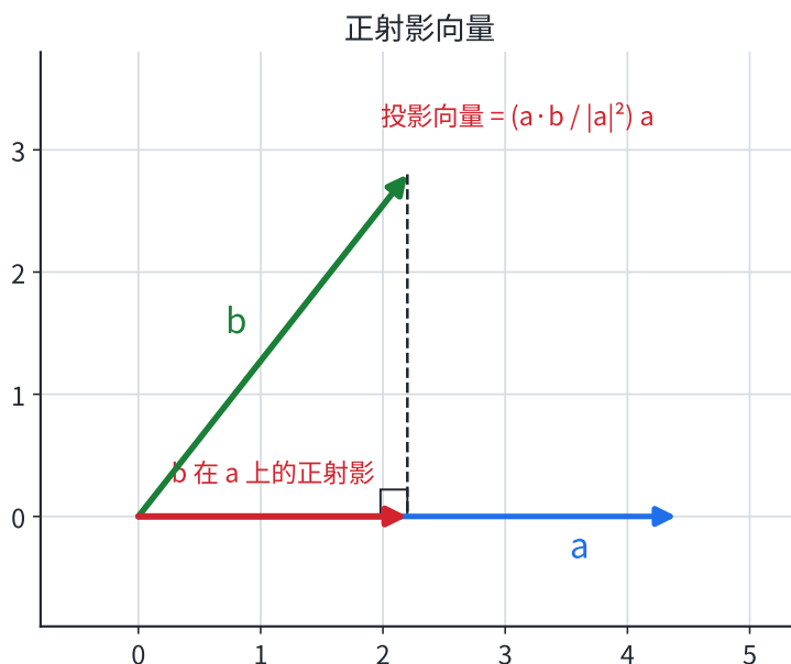
圖 3-4： \vec{b} 在 \vec{a} 上的正射影。從 \vec{b} 的尖端對 \vec{a} 所在直線作垂線，落點與原點之間沿 \vec{a} 方向的那支紅色向量，即正射影向量 \left( \frac{\vec{a} \cdot \vec{b}}{|\vec{a}|^2} \right) \vec{a} 。
