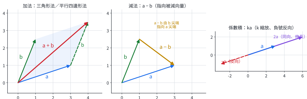
圖 3-1：左——加法（三角形法／平行四邊形法）， \vec{a} + \vec{b} 是平行四邊形的對角線；中——減法 \vec{a} - \vec{b} 由 \vec{b} 的尖端指向 \vec{a} 的尖端；右——係數積 k\vec{a} 沿 \vec{a} 方向縮放，負號則反向。
