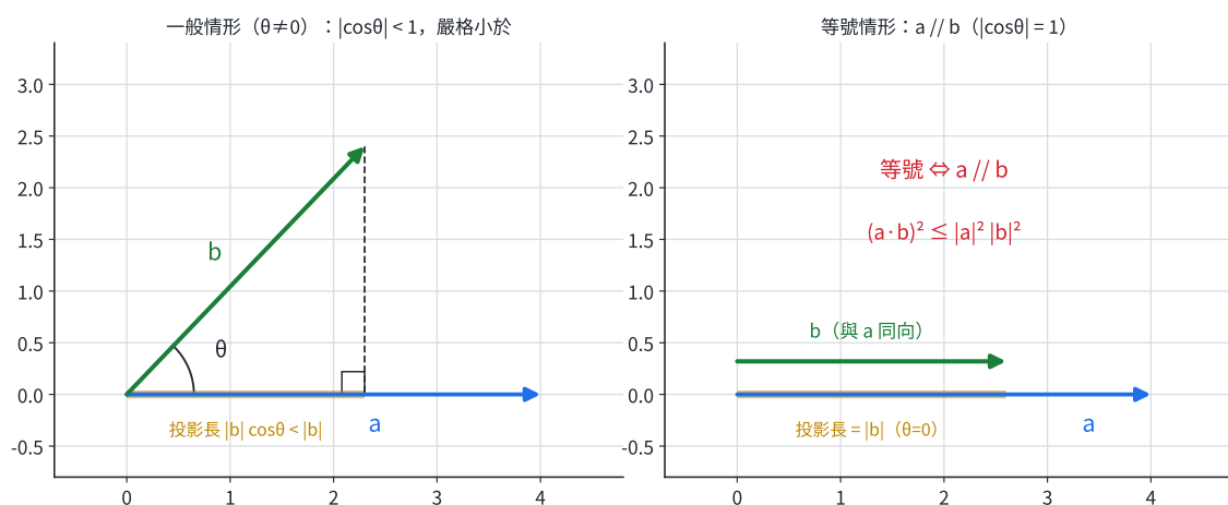
圖 3-6：柯西不等式的幾何意義。左——當 \vec{a} 、 \vec{b} 夾角 \theta \neq 0 時， \vec{b} 在 \vec{a} 上的投影長 |\vec{b}|\cos\theta 嚴格小於 |\vec{b}| （因 |\cos\theta| < 1 ），故 (\vec{a} \cdot \vec{b})^2 < |\vec{a}|^2 |\vec{b}|^2 ；右——當 \vec{a} \parallel \vec{b} ( \theta = 0 ) 時投影長等於 |\vec{b}| ，不等式取等號。柯西不等式正是「 |\cos\theta| \leq 1 」的代數化身。
